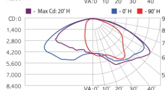
СКУ 150-04У1
