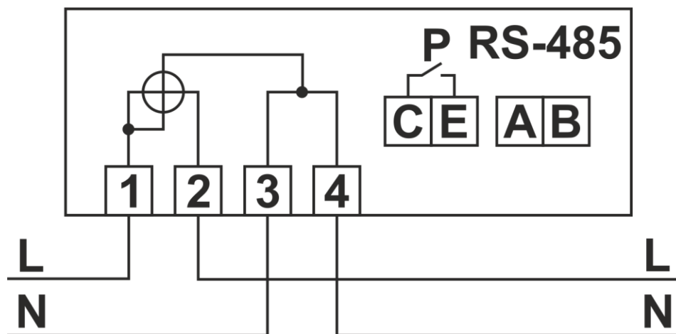
Рис. 1. Схема подключения счётчика
